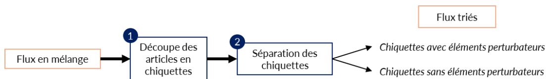
Figure 33 : Schéma du fonctionnement du déliissage sur chiquettes
