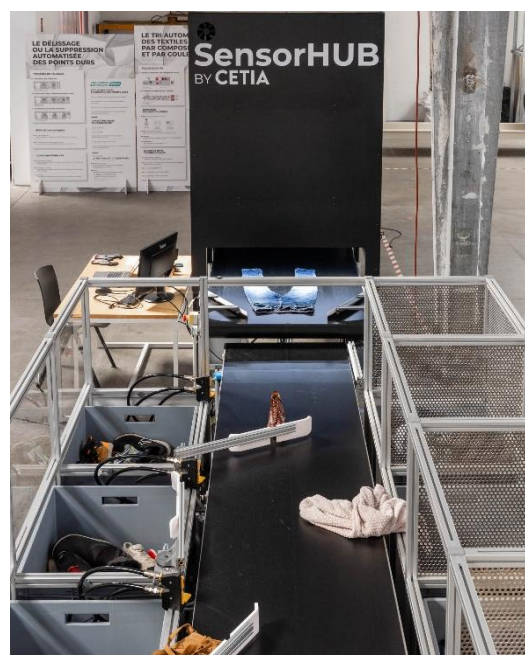
Figure 17 : Cellule SensorHUB Source : CETIA
